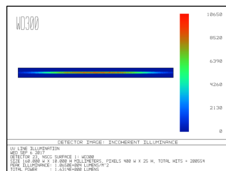
照度分布
